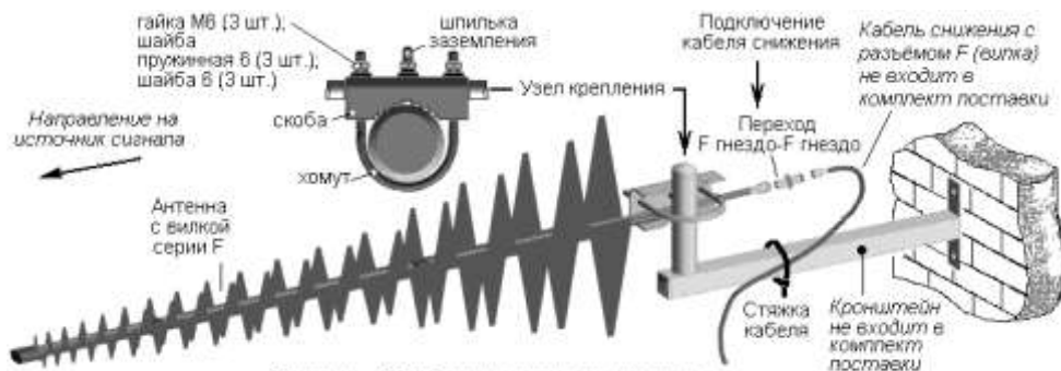
Рисунок - Общий вид и установка антенны
